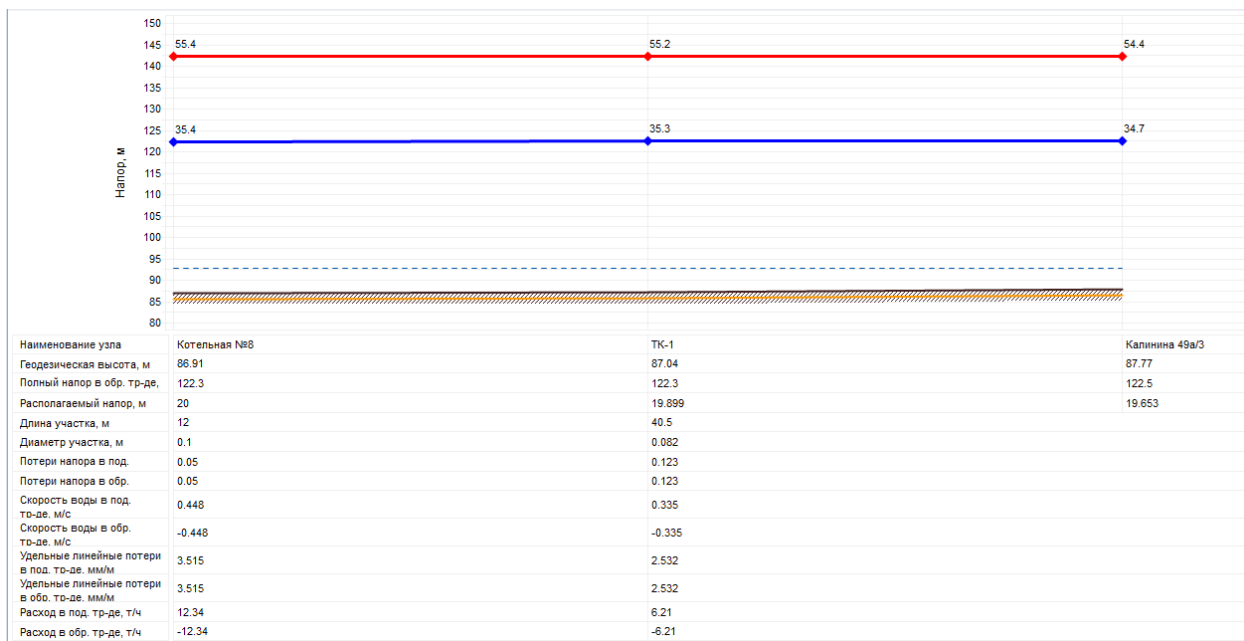
Рисунок 7. Пьезометрический график №8 г. Зерноград, ул. Белинского, 3д
