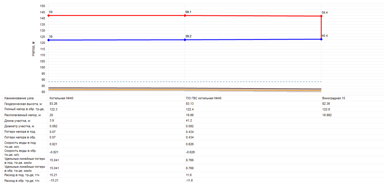
Рисунок 10. Пьезометрический график №40 г. Зерноград, ул. Виноградная, 15
