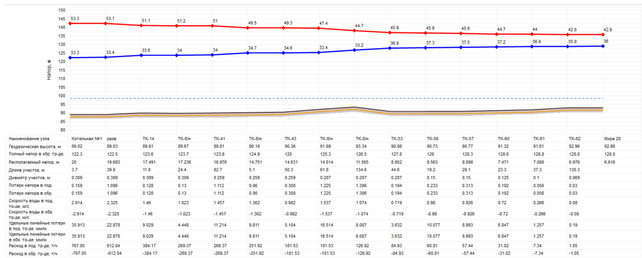
Рисунок 1. Пьезометрический график №1 г. Зерноград, ул. Чкалова, 17д
